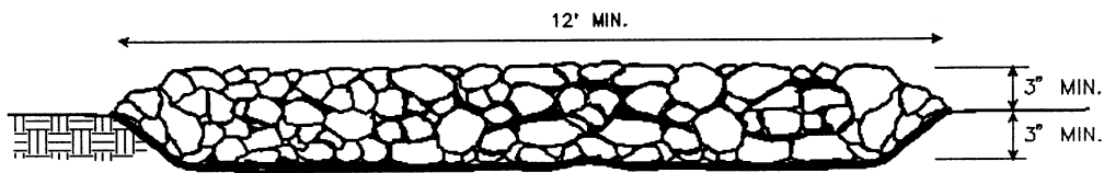
SECTION A-A
